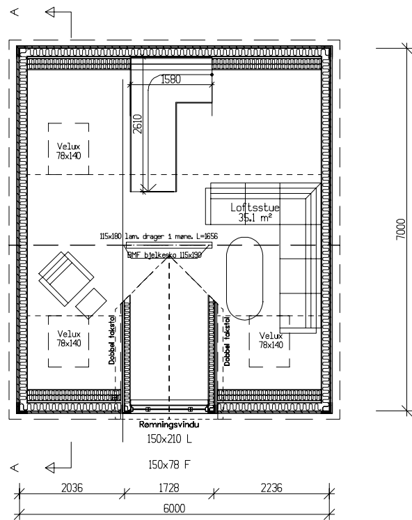
Loftsplan Bra=23,9m²
