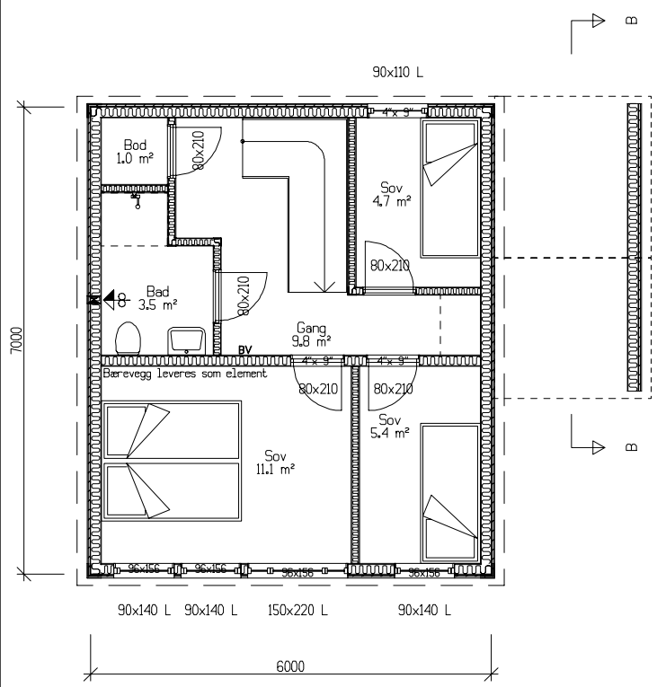
Plan 2. etasje. Bra=37,9m²
