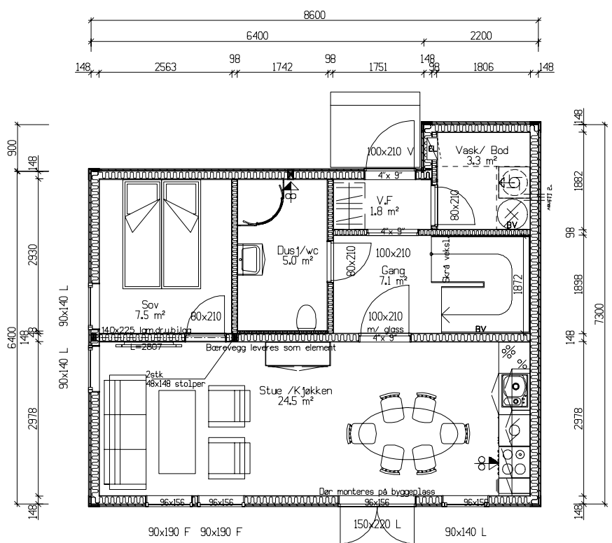
Plan 1. etasje. Bra=51,9m²
