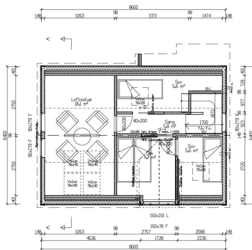
Loftsplan Bra=32,5m²
