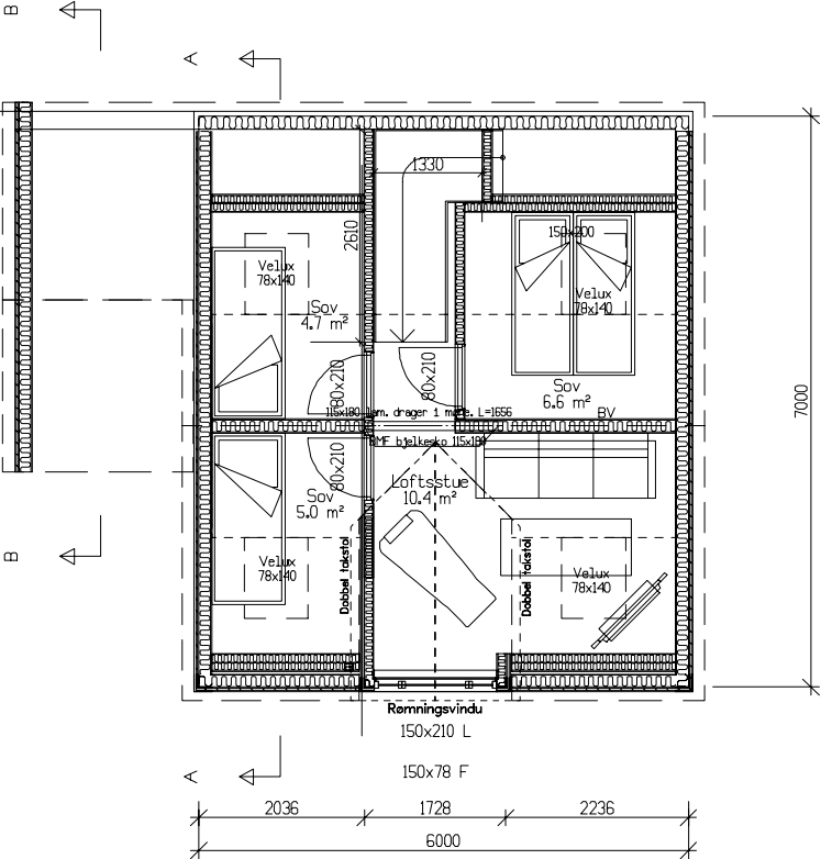
Loftsplan Bra=23,9m²
