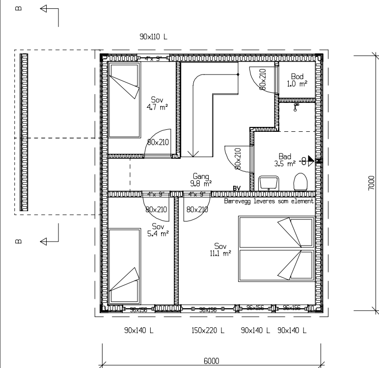
Plan 2. etasje. Bra=37,9m²
