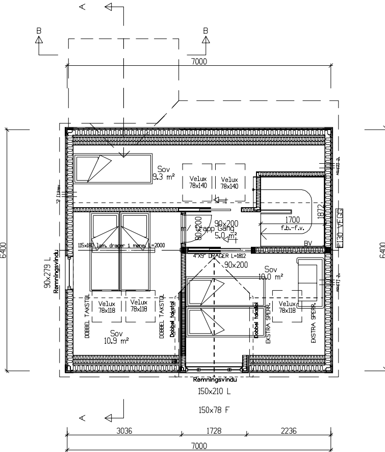
Loftsplan Bra=26,6m²
