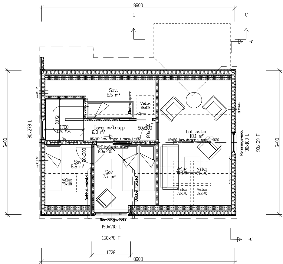
Loftsplan Bra=35,1m²
