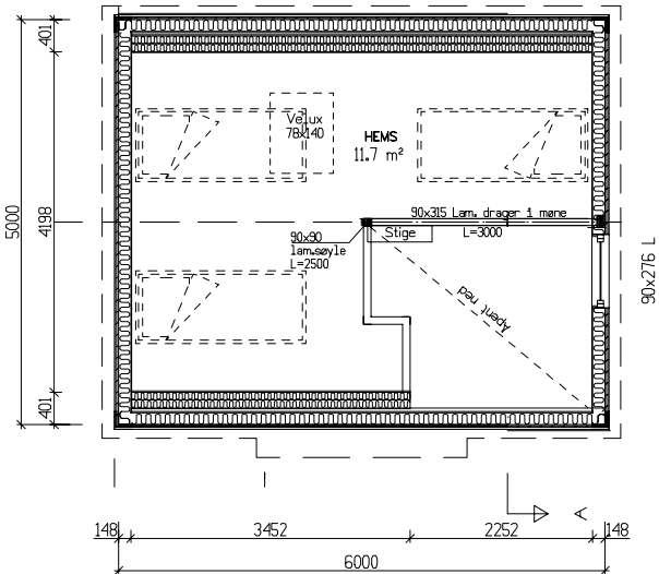
Hems Bra=11,7m²
