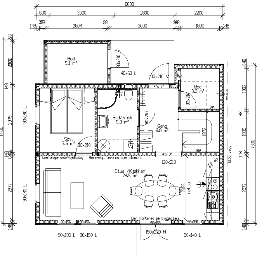
Plan 1. etasje. Brutto=65,5m² / Bra=57,6m²
