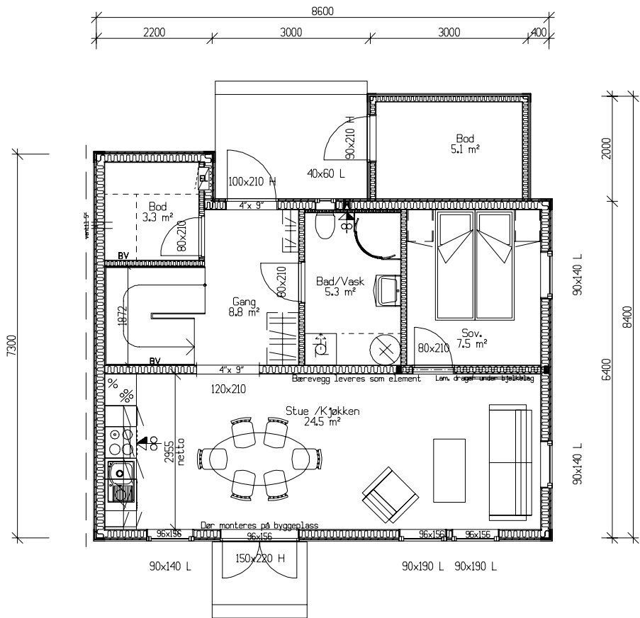
Plan 1. etasje. Brutto=65,5m² / Bra=57,6m²
