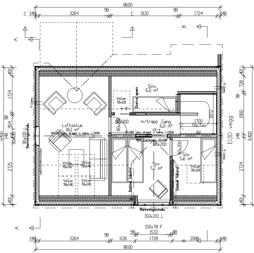
Loftsplan Bra=32,5m²
