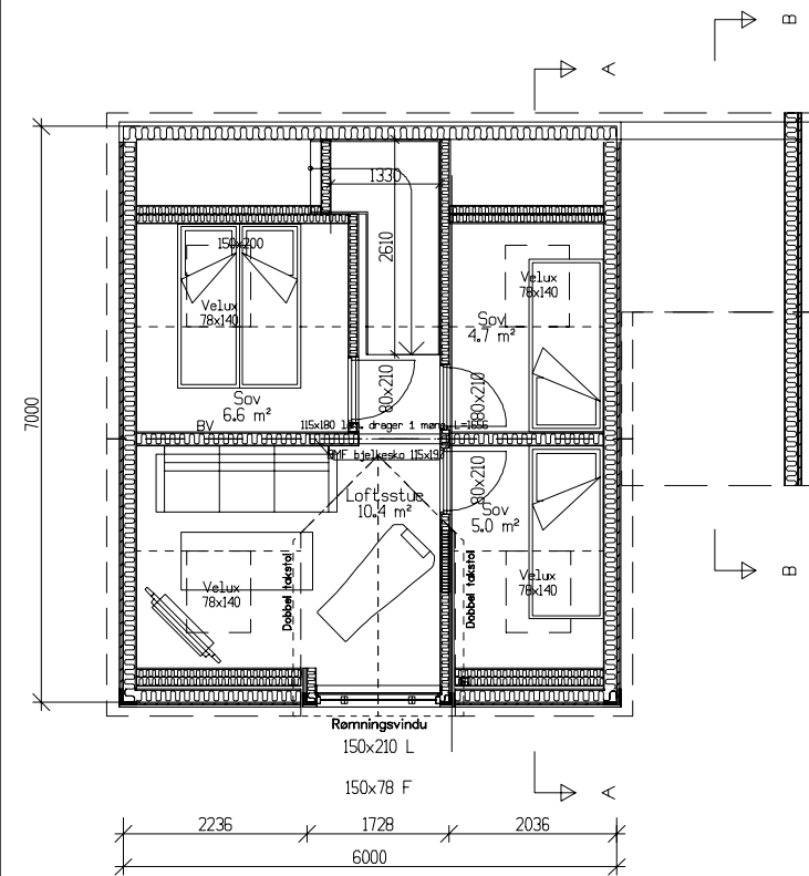
Loftsplan Bra=23,9m²
