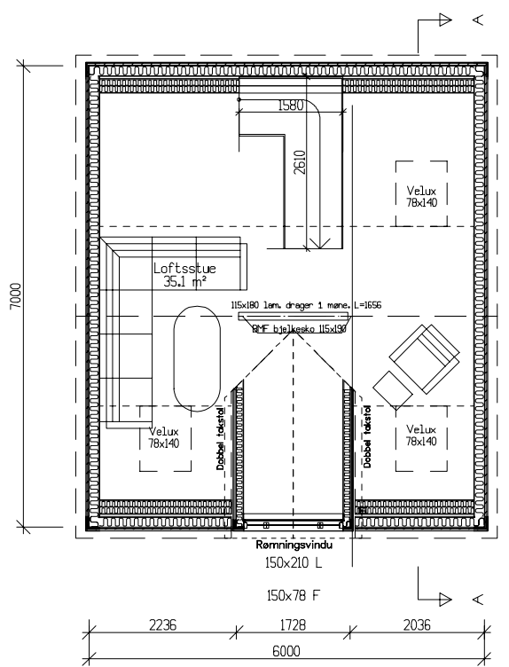
Loftsplan Bra=23,9m²
