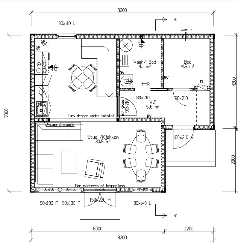
Plan 1. etasje. BYA=52,9m² / BRA=46,3m²
