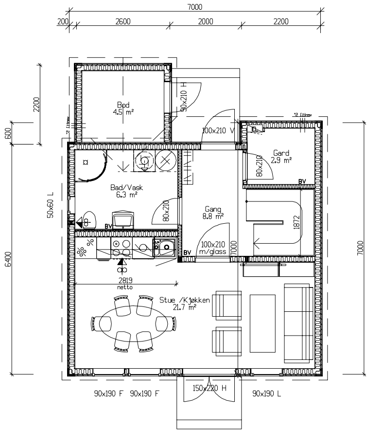
Plan 1. etasje. Brutto=53,7m² / Bra=47,2m²
