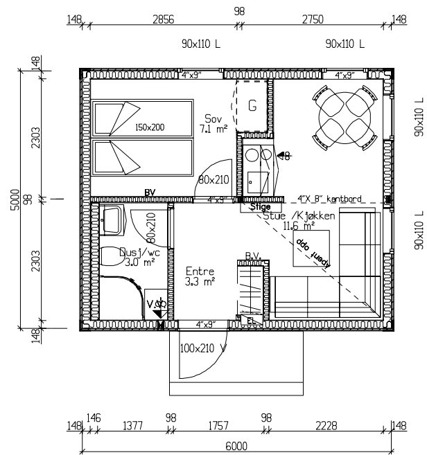
Plan 1. etasje. Brutto=31,2m²/Bra=26,6m²
