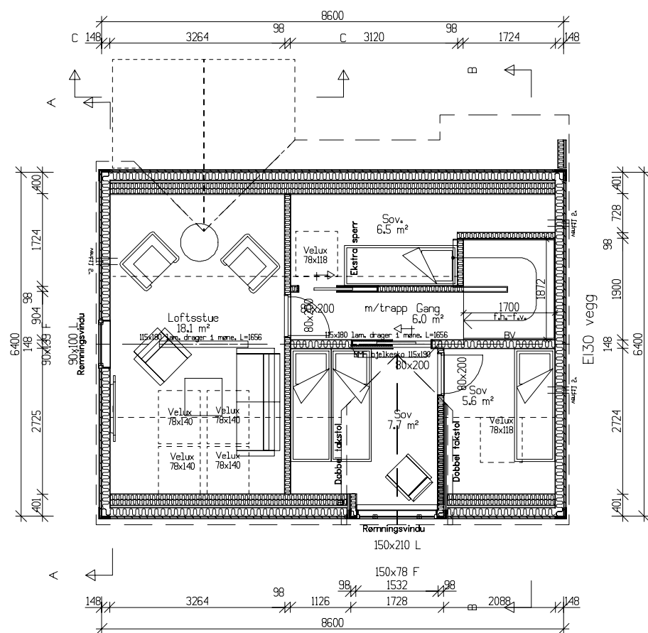
Loftsplan Bra=32,5m 2
