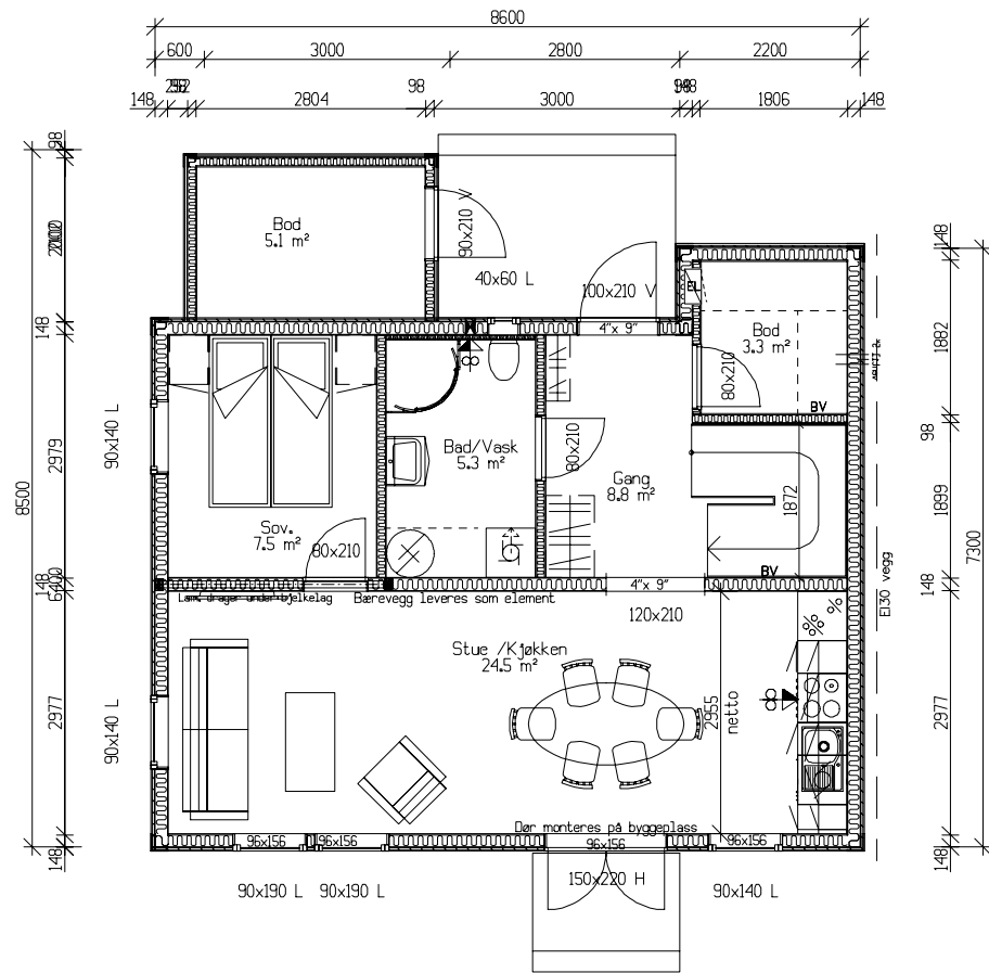
Plan 1. etasje. Brutto=65,5m 2 / Bra=57,6m 2
