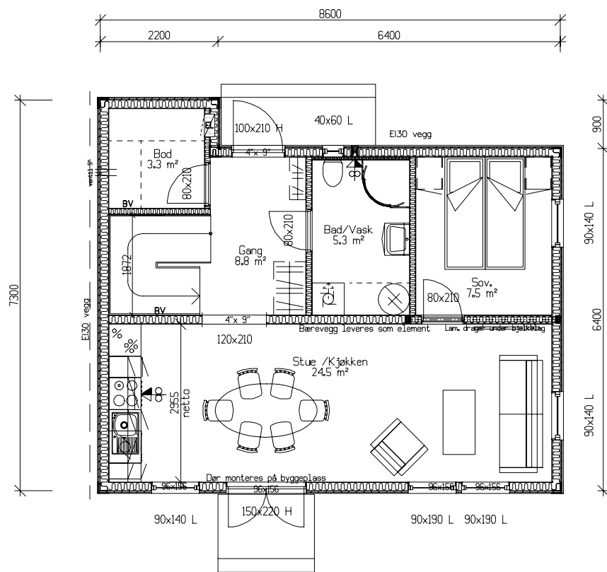
Plan 1. etasje. Brutto=58,7m 2 / Bra=51,9m 2
