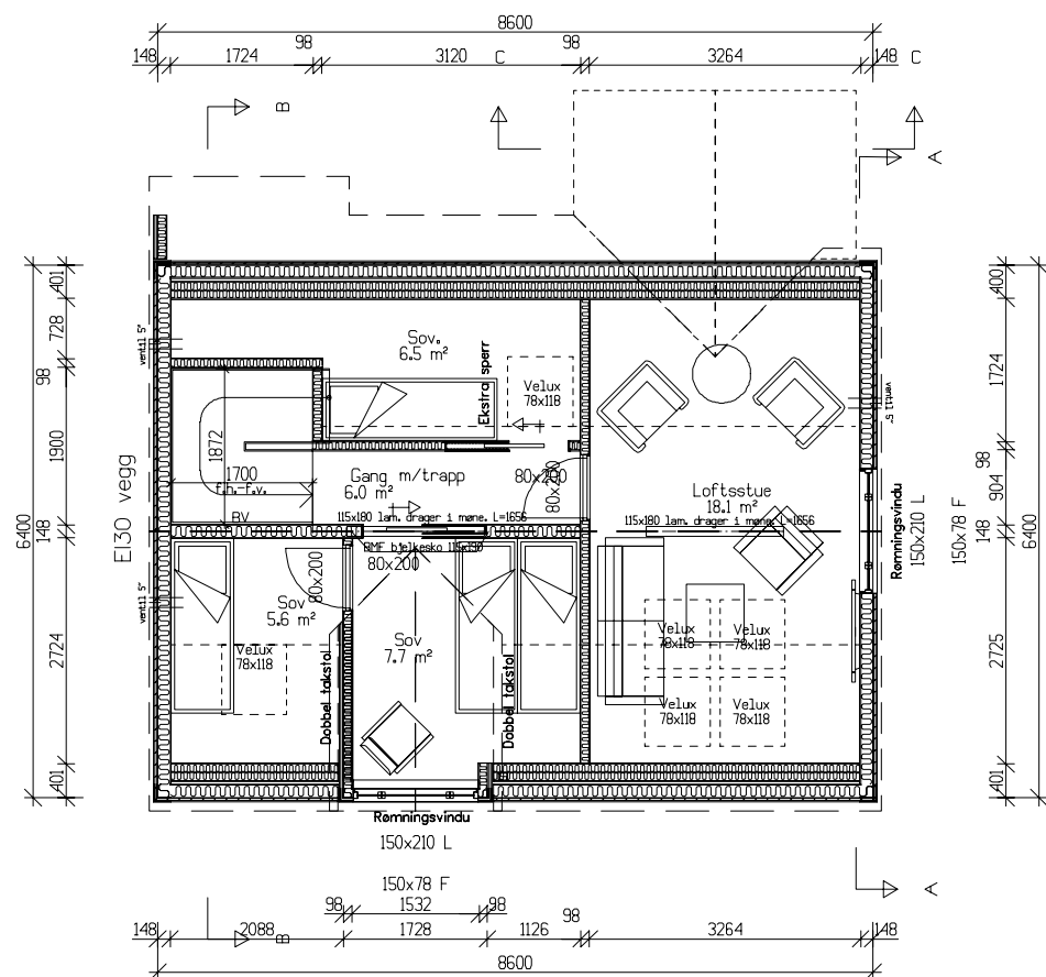
Loftsplan Bra=32,5m 2
