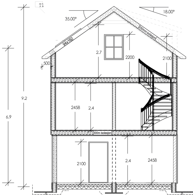
Snitt A-A
