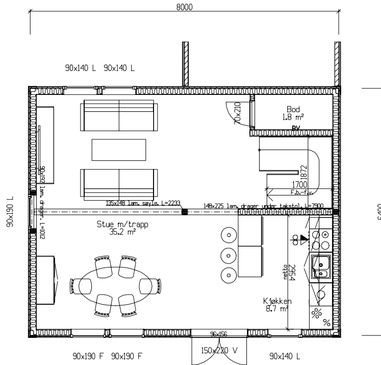
Plan 2. etasje. Bra=46,7m 2
