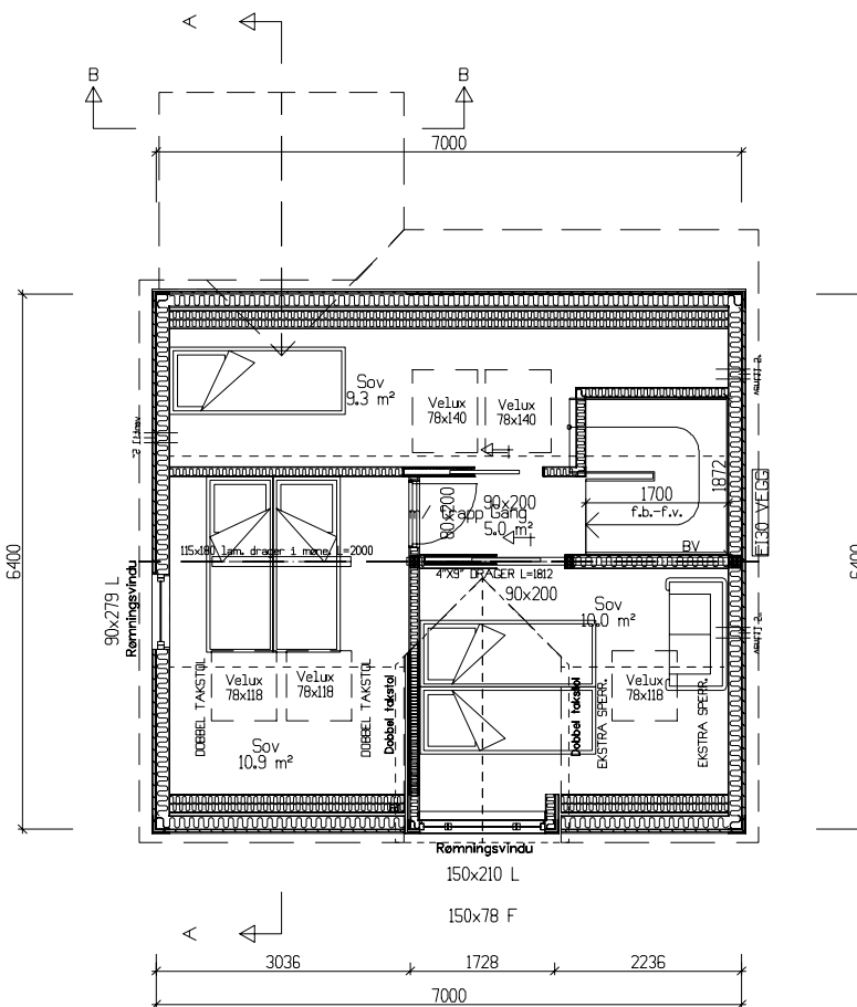
Loftsplan Bra=26,6m 2
