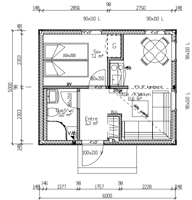
Plan 1. etasje. Brutto=31,2m 2 /Bra=26,6m 2
