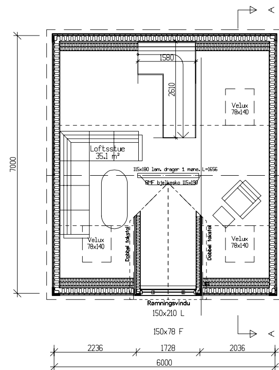
Loftsplan Bra=23,9m 2
