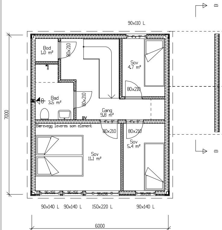
Plan 2. etasje. Bra=37,9m 2
