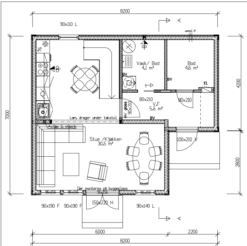
Plan 1. etasje. BYA=52,9m 2 / BRA=46,3m 2
