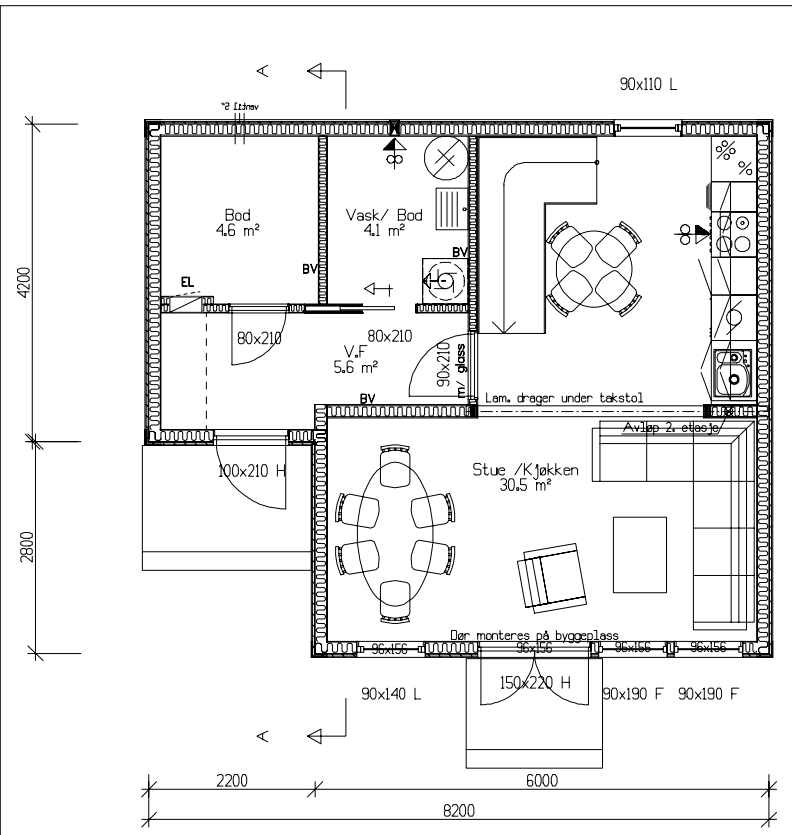
Plan 1. etasje. BYA=52,9m 2 / BRA=46,3m 2
