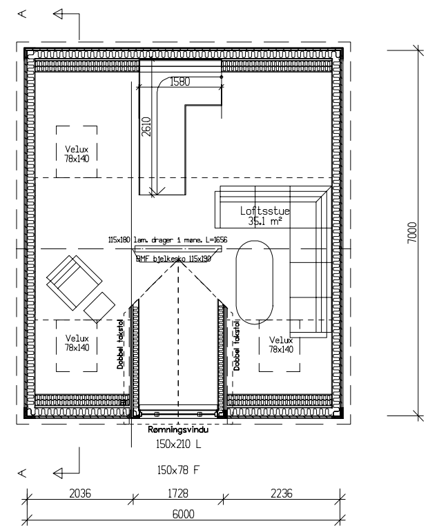
Loftsplan Bra=23,9m 2
