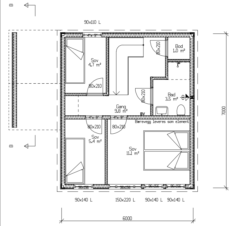
Plan 2. etasje. Bra=37,9m 2
